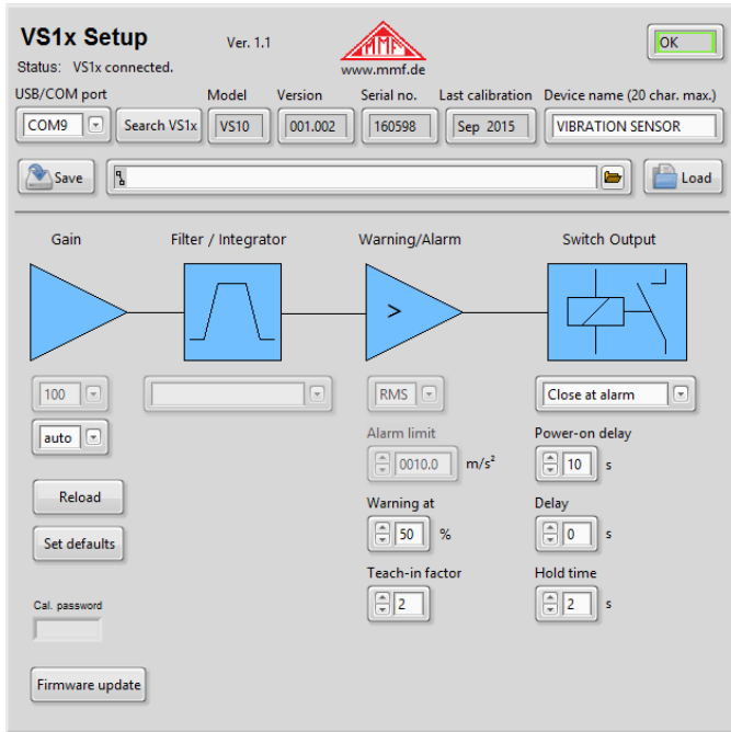
Bild 2: Parametrierprogramm
